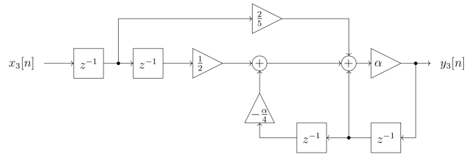
Abbildung 4: LTI-System.
