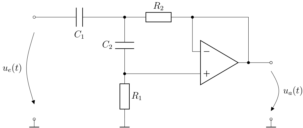
Abbildung 7: Aktives Filter
