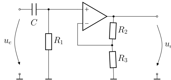
Abbildung 6: Analoges Filter
