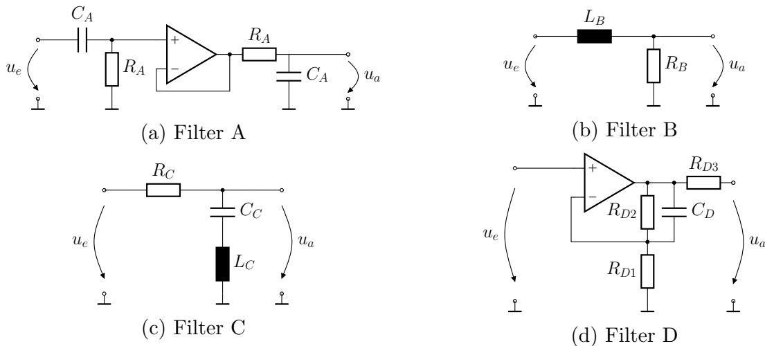
Abbildung 5: Analoge Filter
