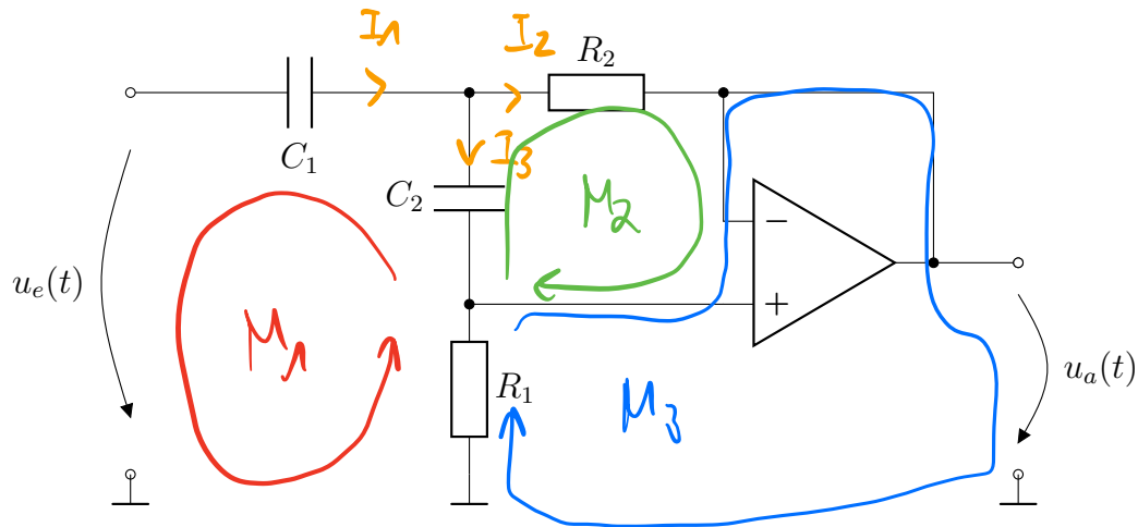
Abbildung 7: Aktives Filter
