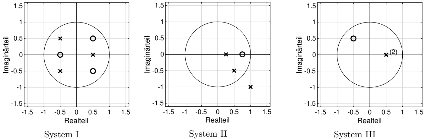
Abbildung 9: Pol-Nullstellen-Diagramme.
