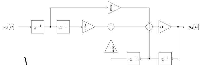
Abbildung 4: LTI-System.
