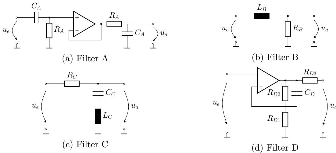
Abbildung 5: Analoge Filter
