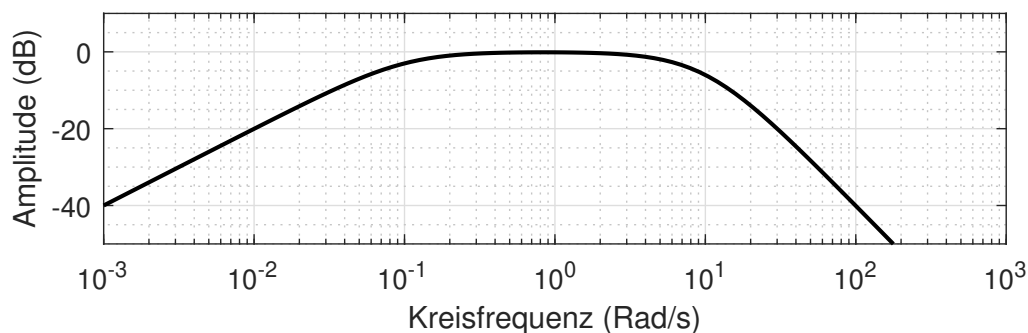
Abbildung 8: Amplitudengang
