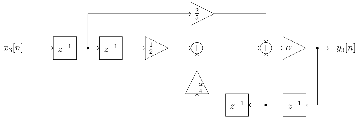
Abbildung 4: LTI-System.
