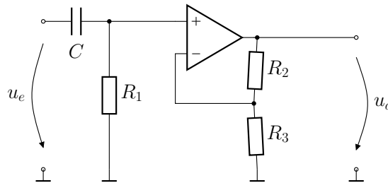
Abbildung 6: Analoges Filter
