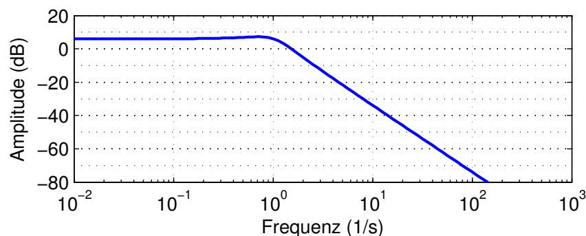
Abbildung 7: Amplitudengang
