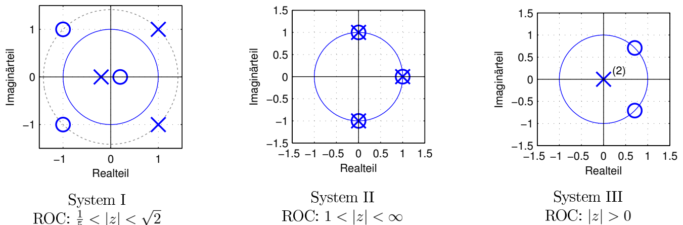
Abbildung 8: Pol-Nullstellen-Diagramme.
