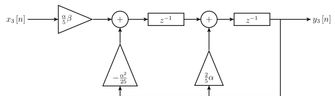
Abbildung 4: LTI-System.
