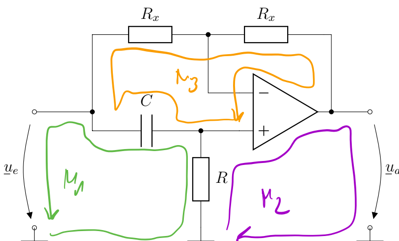
Abbildung 6: Schaltung C
