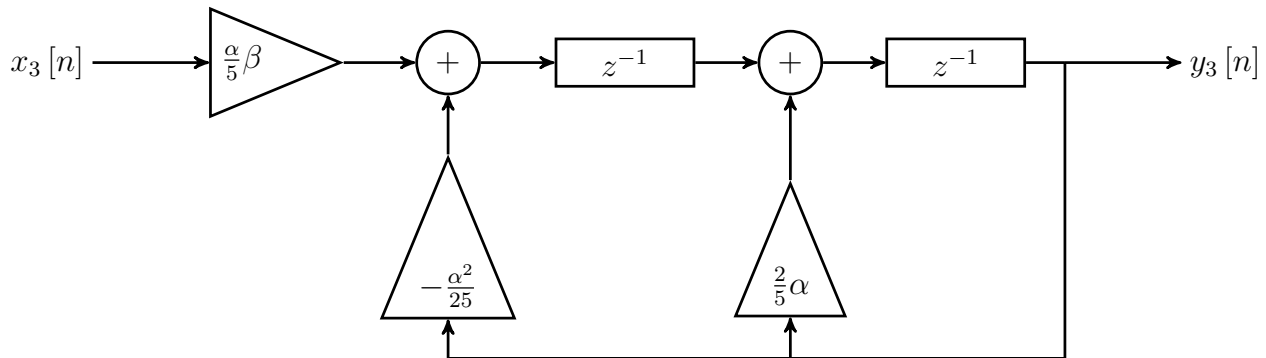
Abbildung 4: LTI-System.
