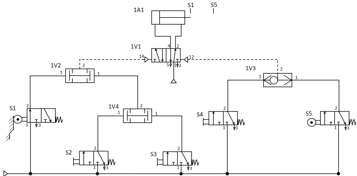
Abbildung 9: Pneumatisches Steuersystem
