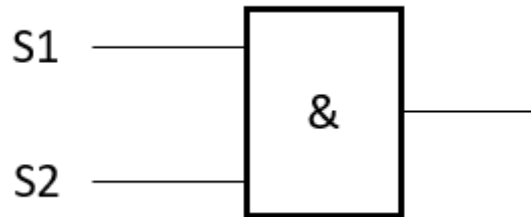
Abbildung 8: Realisierung einer Zwei-Hand-Betätigung
