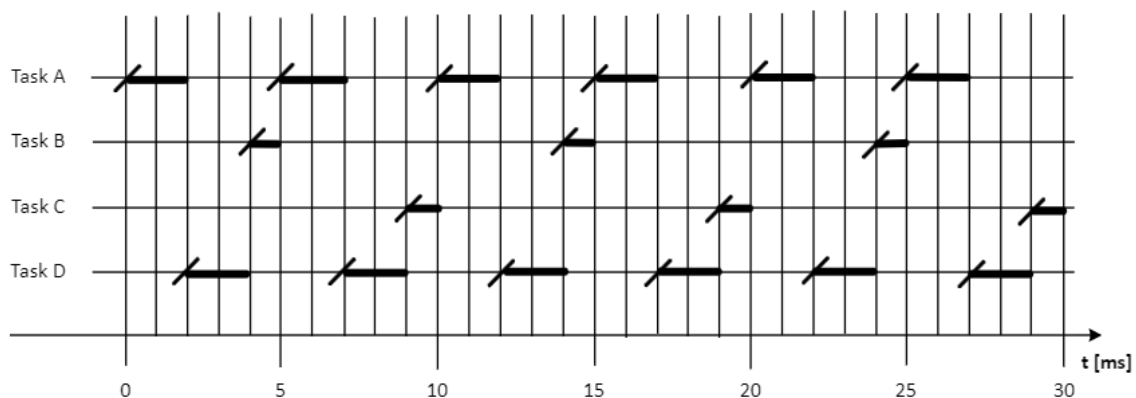
Abbildung 5: Ist-Ablauf der Tasks A, B, C und D (feste Prioritäten)
