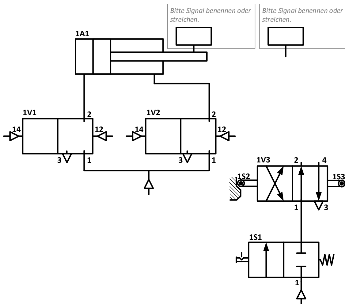
Abbildung 8: Pneumatische Steuerung
