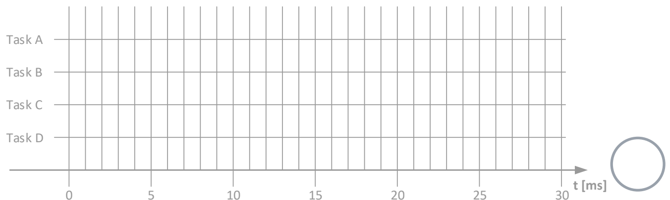
Abbildung 5: Ist-Ablauf der Tasks A, B, C und D (Restantwortzeit-Scheduling)
