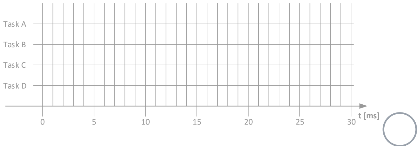
Abbildung 4: Ist-Ablauf der Tasks A, B, C und D (Scheduling mit festen Prioritäten)
