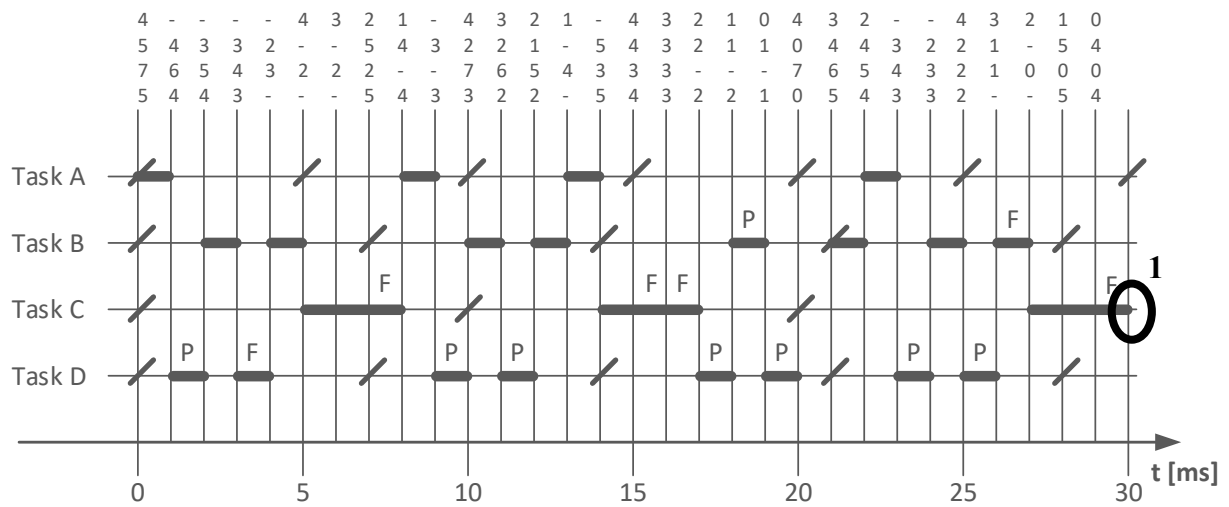
Abbildung 3: Ist-Ablauf der Tasks A, B, C und D (Kleinster Spielraum)
