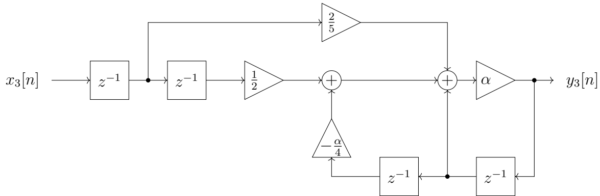
Abbildung 4: LTI-System.
