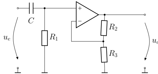
Abbildung 6: Analoges Filter
