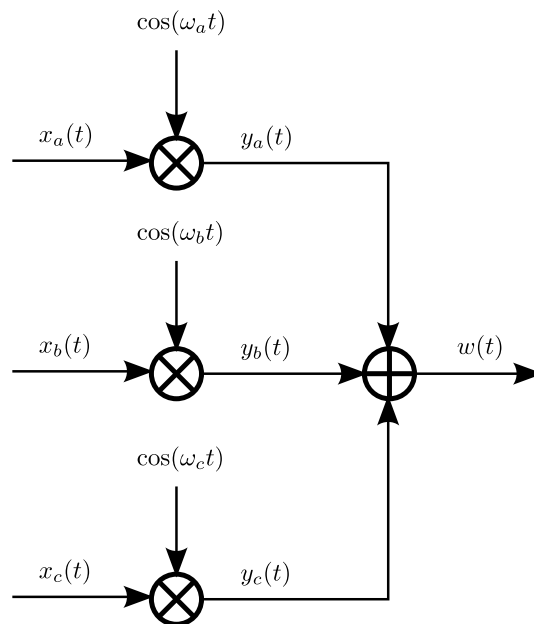
Abbildung 1: Frequenzmultiplex unter Verwendung sinusförmiger Amplitudenmodulation.
