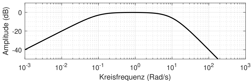
Abbildung 8: Amplitudengang
