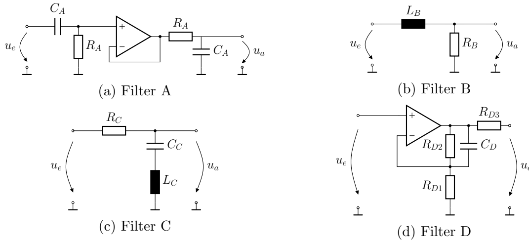
Abbildung 5: Analoge Filter
