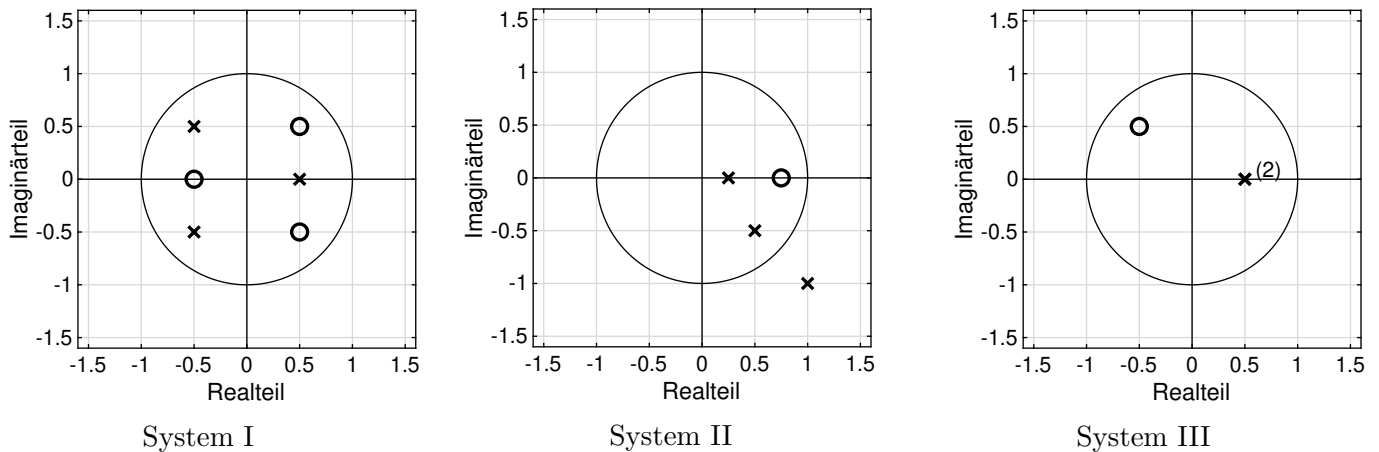
Abbildung 9: Pol-Nullstellen-Diagramme.
