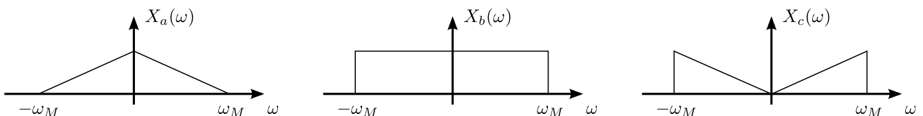
Abbildung 2: Bandbegrenzte Spektren der Siganle der Kanäle a, b und c.
