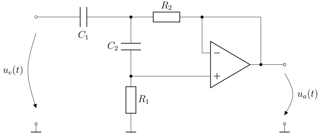
Abbildung 7: Aktives Filter
