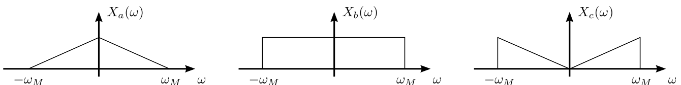
Abbildung 2: Bandbegrenzte Spektren der Signale der Kanäle a, b und c.
