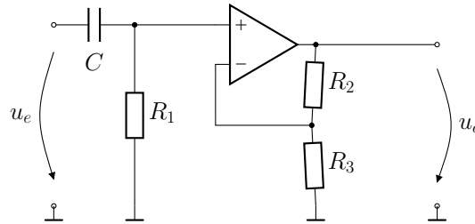
Abbildung 6: Analoges Filter
