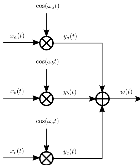
Abbildung 1: Frequenzmultiplex unter Verwendung sinusförmiger Amplitudenmodulation.
