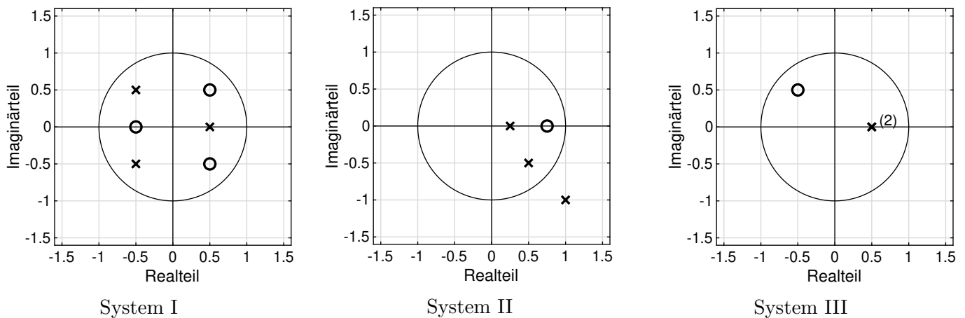
Abbildung 9: Pol-Nullstellen-Diagramme.
