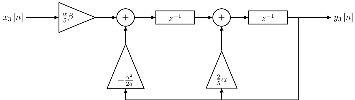
Abbildung 4: LTI-System.
