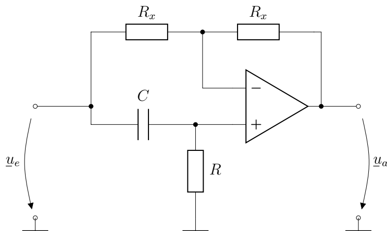
Abbildung 6: Schaltung C
