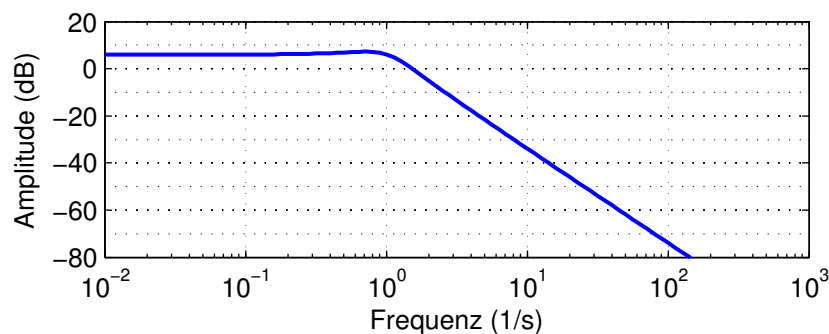
Abbildung 7: Amplitudengang
