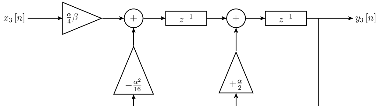
Abbildung 5: LTI-System.
