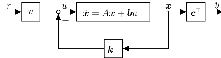
Abbildung 5: Blockschaltbild der Strecke mit Regler und Vorfilter.
