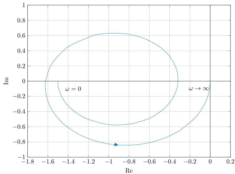
Abbildung 4: Ortskurve der Regelstrecke G .
