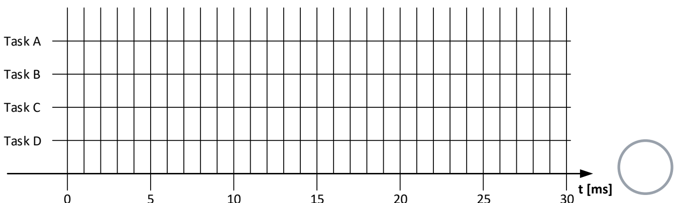
Abbildung 4: Ist-Ablauf der Tasks A, B, C und D (Verfahren der kleinsten Restantwortzeit)
