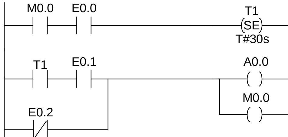
Abbildung 8: SPS-Programm in KOP
