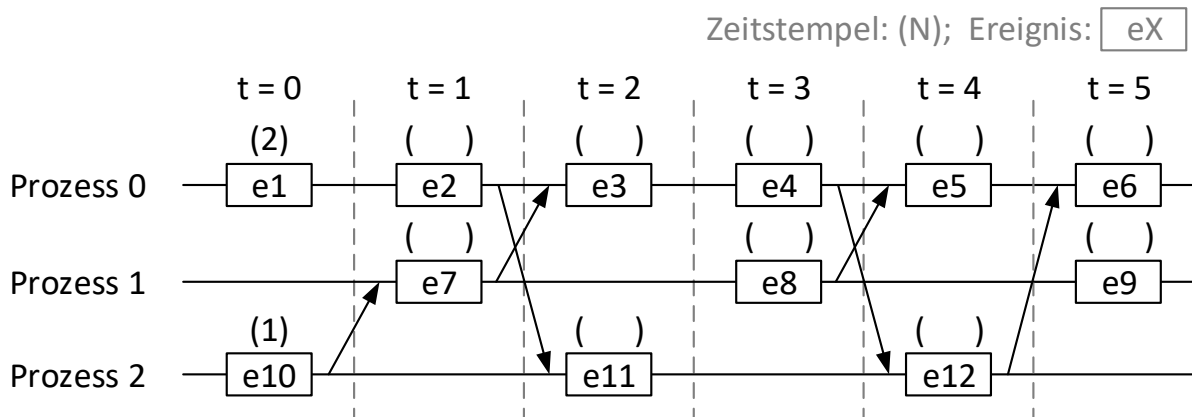
Abbildung 10: Lamport-Uhr mit drei Prozessen
