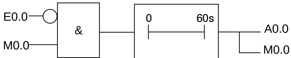
Abbildung 10: SPS-Programm in FUP
