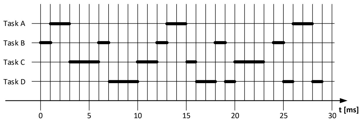
Abbildung 11: Ist-Ablauf der Tasks A, B, C und D (feste Prioritäten)
