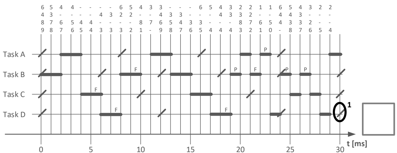
Abbildung 4: Ist-Ablauf der Tasks A, B, C und D (Kleinsten Spielraum)
