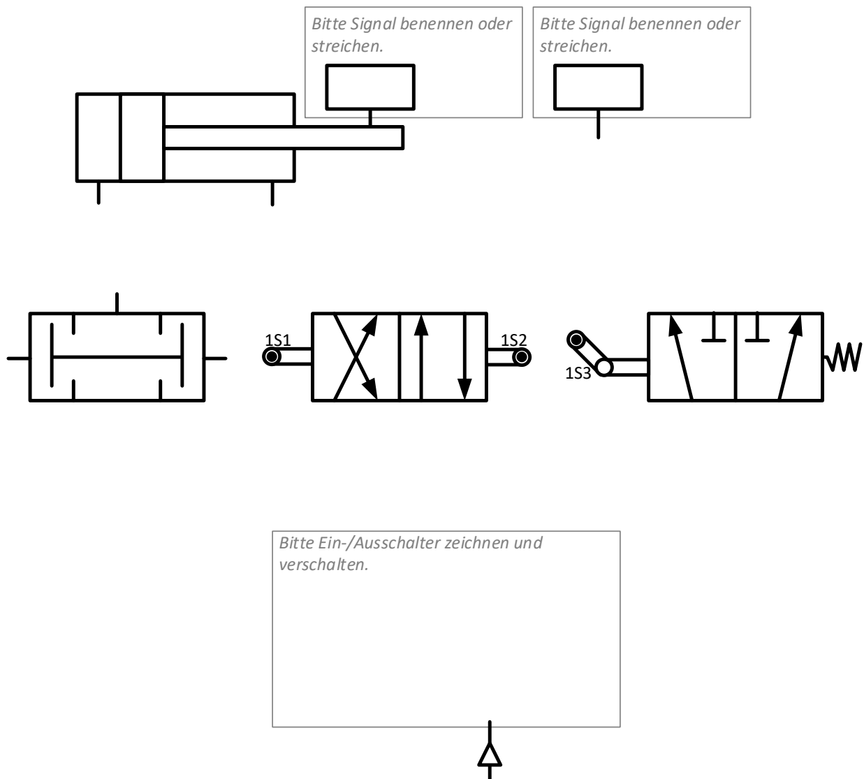
Abbildung 15: Pneumatische Steuerung
