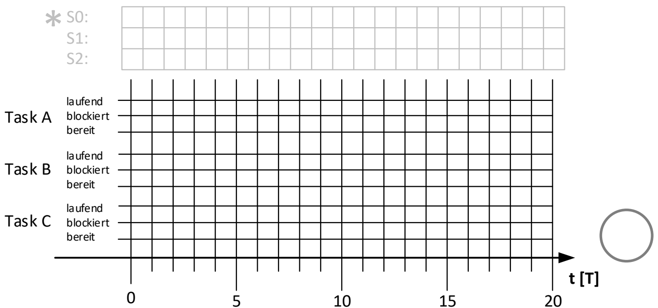
Abbildung 11: Ist-Ablauf der Tasks A, B und C (Priority Inheritance)
